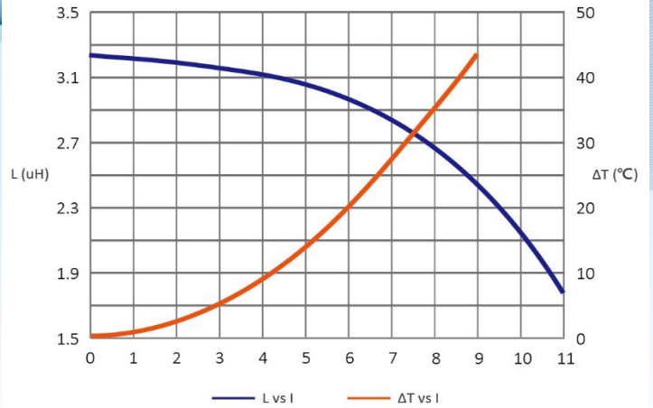
SAR7050MT3R3-M
