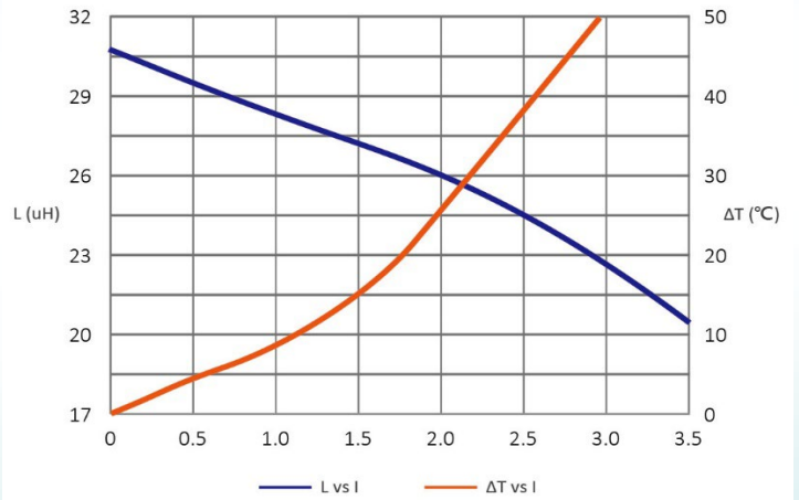
SAR7050MT330-M
