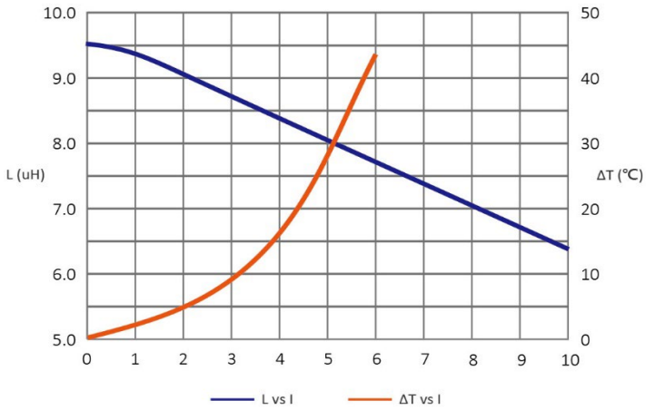
SAR7050MT100-M
