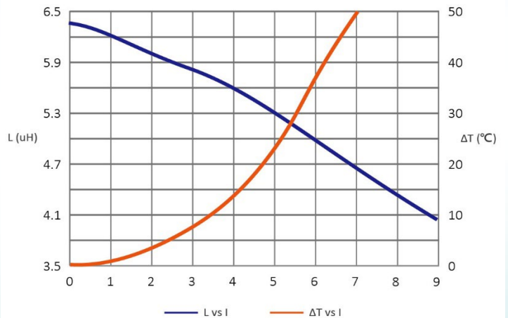
SAR7050MT5R6-M
