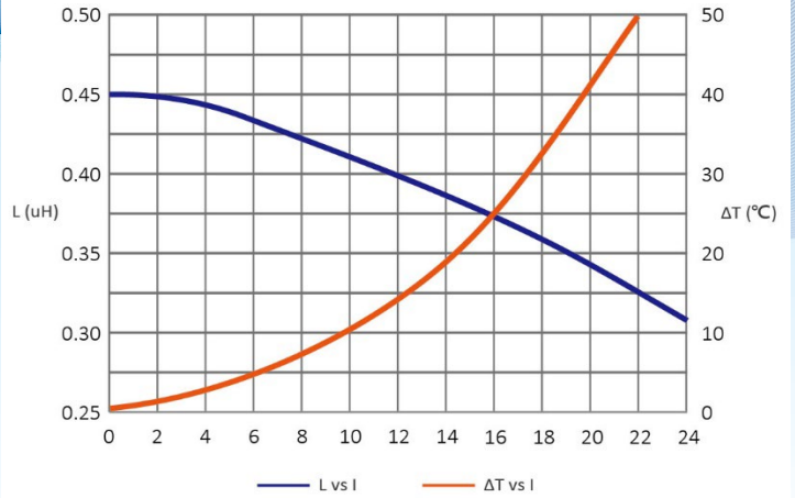
SAR7050MTR47-M
