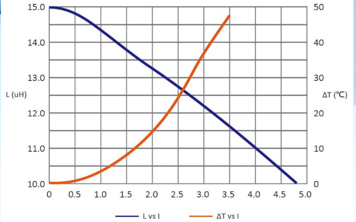
SAR7050MT150-M
