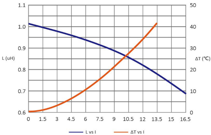
SAR7050MT1R0-M
