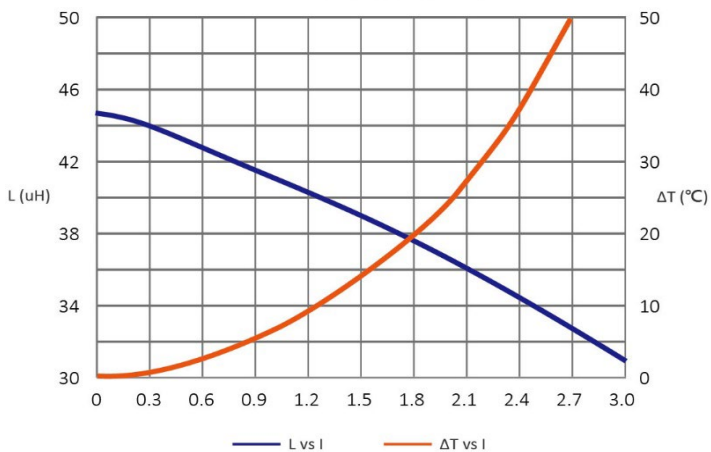
SAR7050MT470-M
